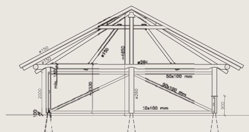
Snit A-A – 1:50
