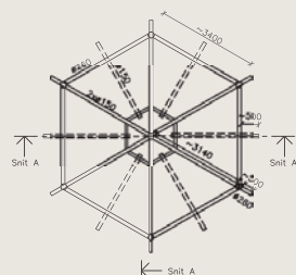
Plan 1:100
