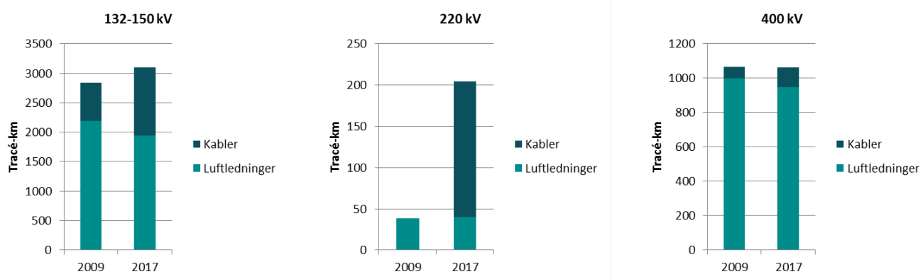
Figur 1 Omfang af kabler og luftledninger i tracé-km inden igangsætning af kabelhandlings- og forskønnelsesplanerne i 2009 og primo 2017.
