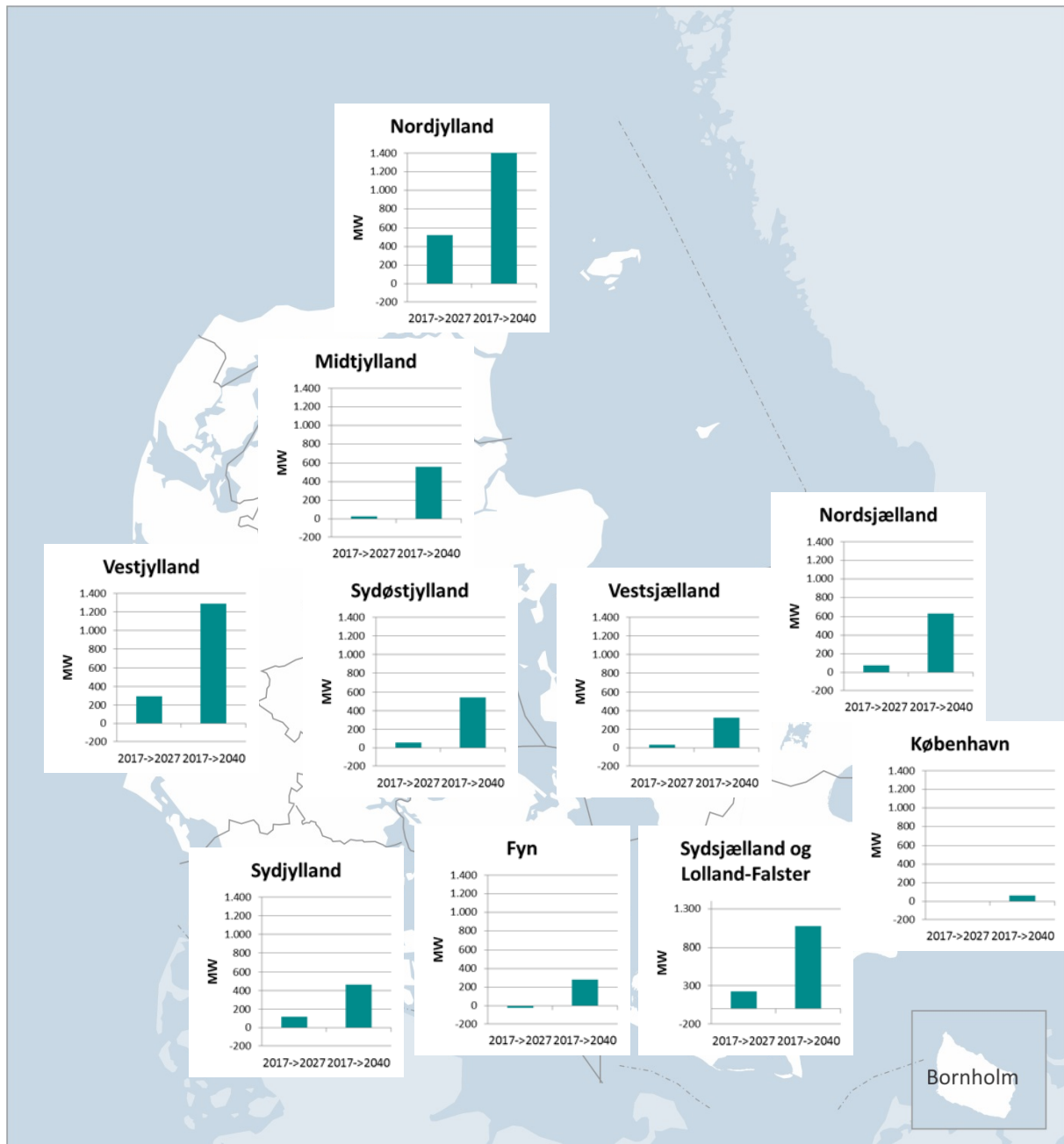
Figur 10 Ændring i installeret effekt fra VE-anlæg fra henholdsvis 2017 til 2027 og 2017 til 2040.
