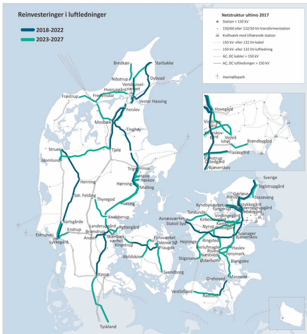
Figur 22 Illustration af reinvesteringsbehovet i eksisterende ledningsanlæg for de kommende 10 år.
